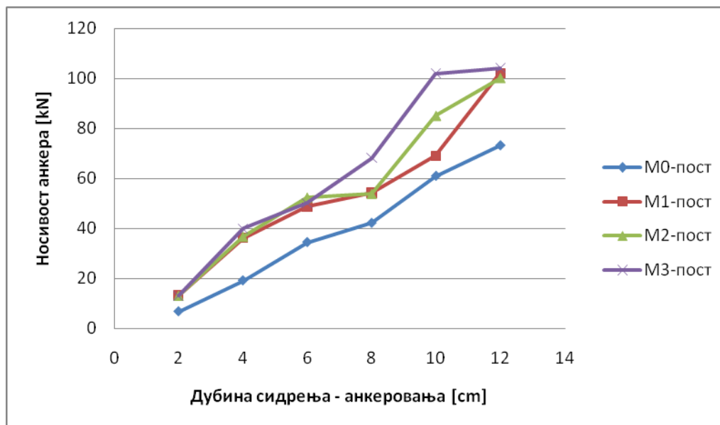
Слика 7.11/3 - Веза носивости анкера на затезање и дубине анкеровања за величину анкера R16 (накнадно уграђени - хемијски анкери)
