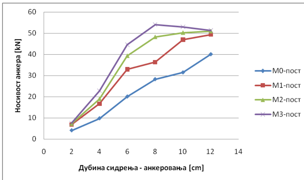
Слика 7.11/1 - Веза носивости анкера на затезање и дубине анкеровања за величину анкера R10 (накнадно уграђени - хемијски анкери)
