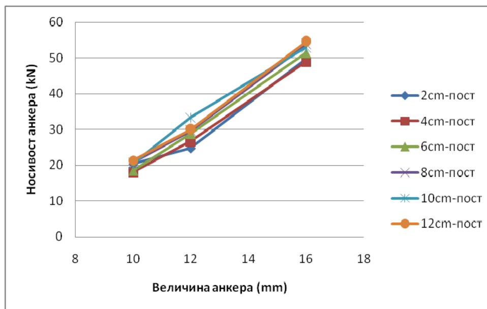
Слика 7.13/4 - Носивост хемијских анкера на смицање у бетону М3
