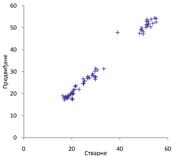
Тренирање 90% резултата
