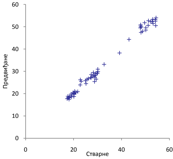
Тренирање 90% резултата
