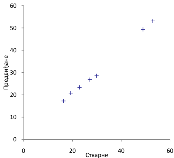
Тестирање 10% резултата
