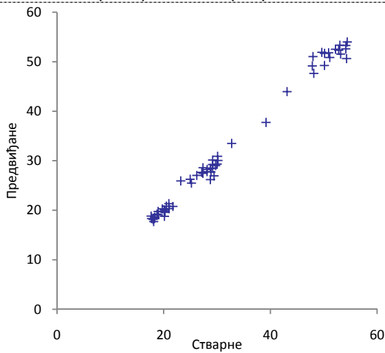
Тренирање 80% резултата
