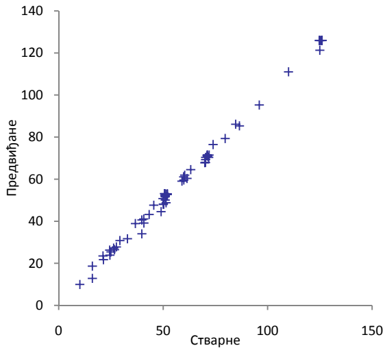
Тренирање 85% резултата
