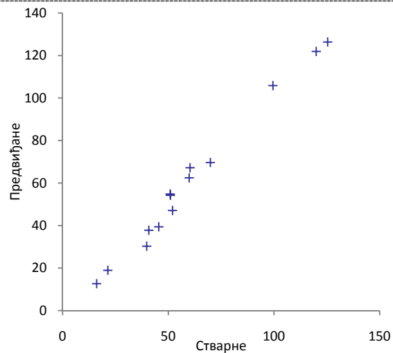
Тестирање 20% резултата
