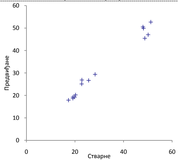
Тестирање 20% резултата
