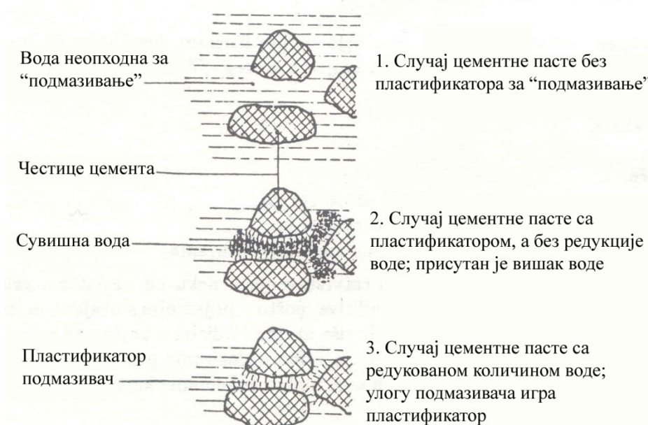
Слика 2.3 - Механизам деловања пластификатора у бетону [4]
