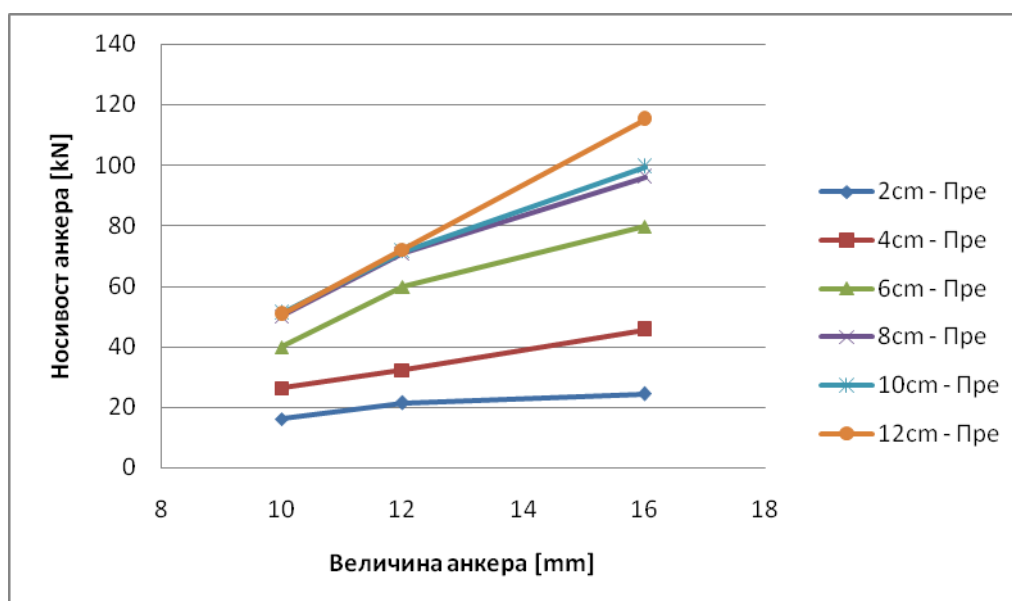
Слика 7.8/2 - Веза носивости анкера на затезање и величине анкера у бетону М1 за различите дубине сидрења - анкеровања (претходно уграђени анкери)
