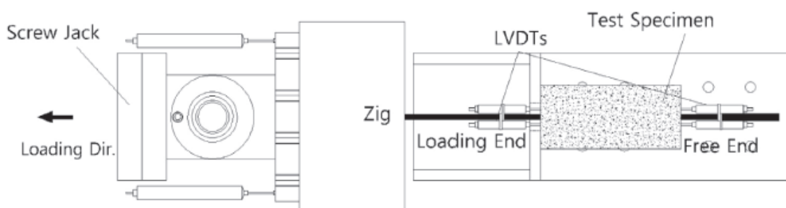
Слика 4.4 - Диспозиција испитивања V.I.Вае и остали [47]
