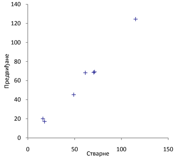
Тестирање 10% резултата
