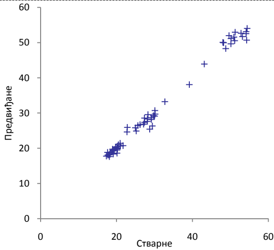
Тренирање 85% резултата
