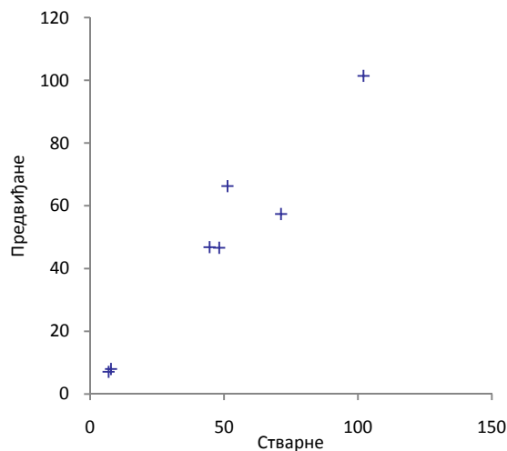
Тестирање 10% резултата
