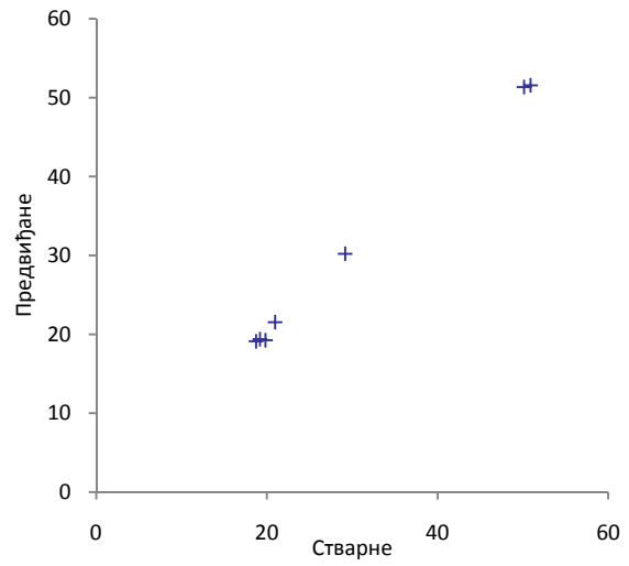
Тестирање 10% резултата
