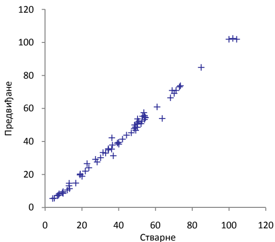
Тренирање 90% резултата
