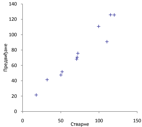
Тестирање 15% резултата
