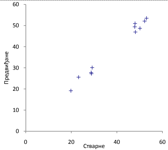
Тестирање 15% резултата
