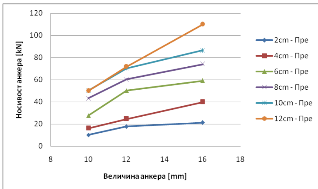
Слика 7.8/1 - Веза носивости анкера на затезање и величине анкера у бетону М0 за различите дубине сидрења - анкеровања (претходно уграђени анкери)
