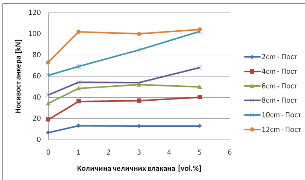
Слика 7.7/3 - Однос носивости анкера и количине челичних влакана за анкер R16
