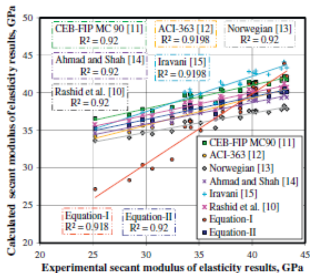
Слика 2.19 -Поређење стварних и рачунских вредности модула еластичности
