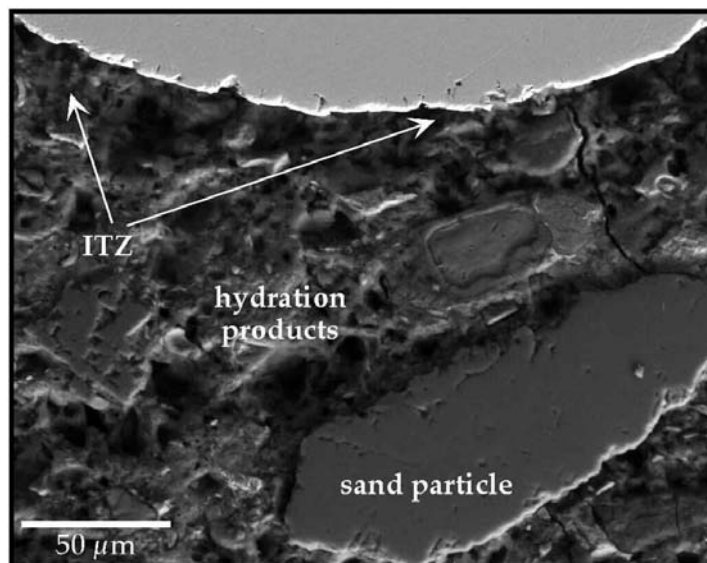
Слика 2.12а -SEM слика транзитне зоне између влакна и цементне матрице
