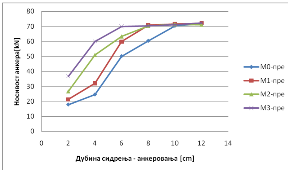
Слика 7.10/2 - Веза носивости анкера на затезање и дубине анкеровања за величину анкера R12 (претходно уграђени анкери)
