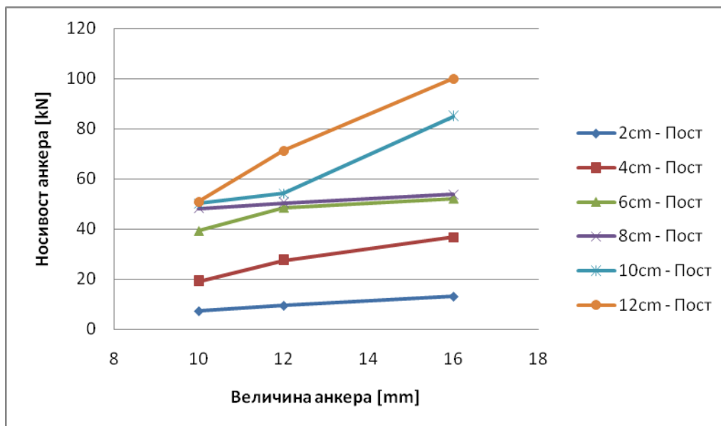
Слика 7.9/3 - Веза носивости анкера на затезање и величине анкера у бетону М2 за различите дубине сидрења - анкеровања (хемијски анкери)
