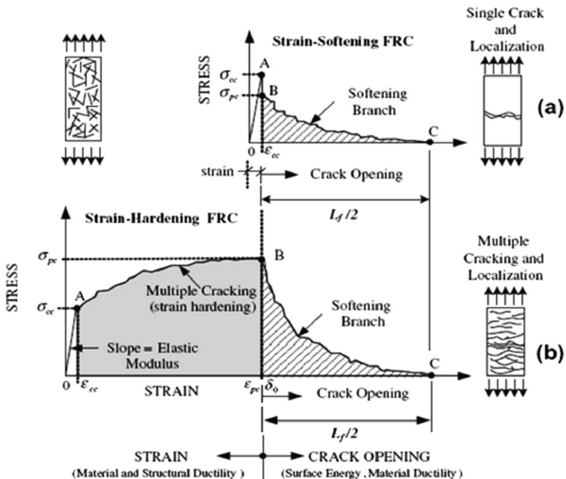
Слика 2.20 - Карактеристични дијаграми напона-дилатација
